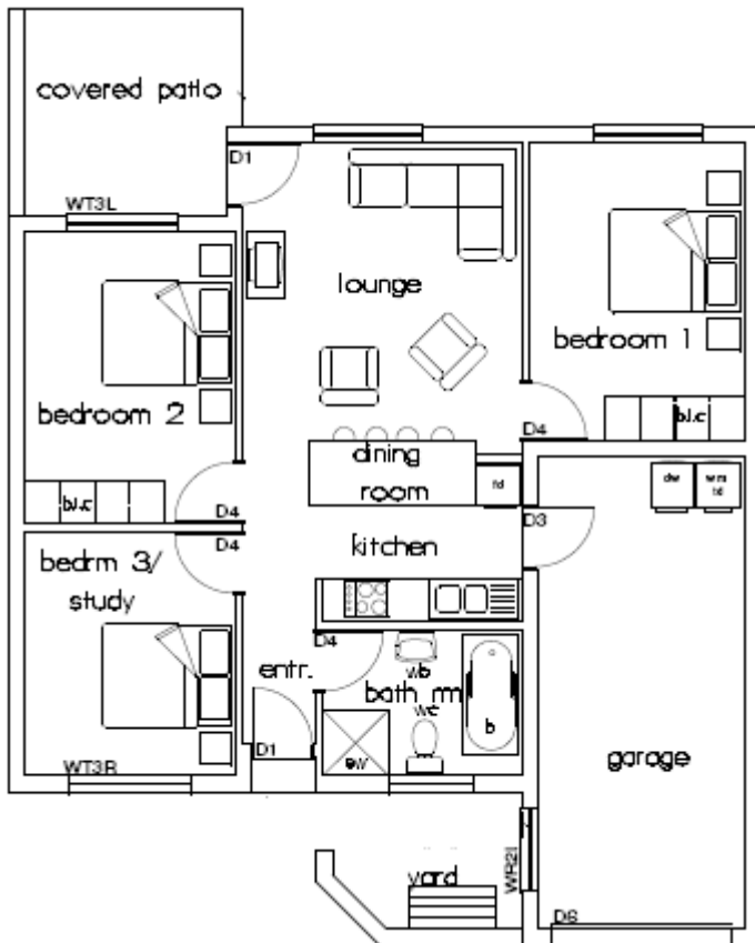
3 Bedroom Type 4
