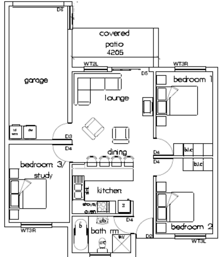
3 Bedroom Type 5
